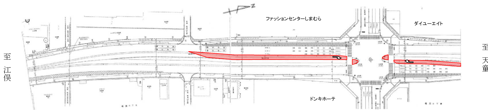
《平面図》
